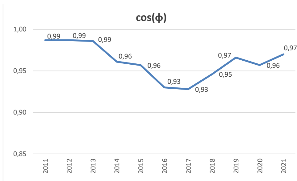
Σχήμα 3-2: Αύξηση και σταθεροποίηση συντελεστή εκμετάλλευσης ηλ. ενέργειας ( \cos\phi ), μετά από επενδύσεις (μέσες ετήσιες τιμές)
