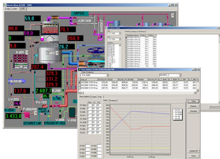
Σχήμα 1-2: Στο εργοστάσιο της LPC, χρησιμοποιούνται σύγχρονα συστήματα για τον έλεγχο των διεργασιών, την βελτίωση της απόδοσης και την πρόληψη ατυχημάτων
