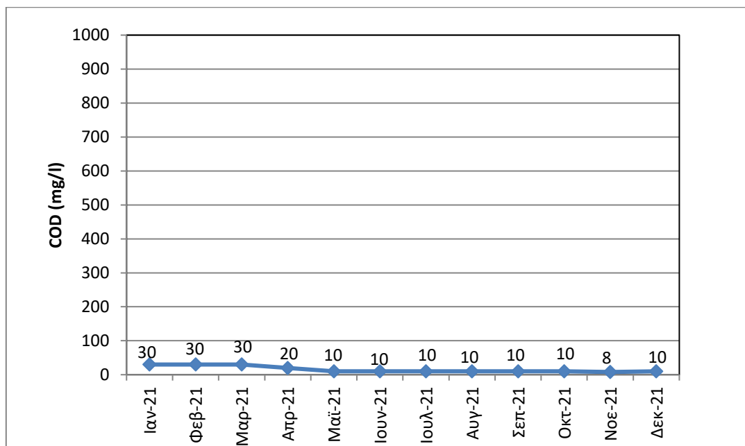
Σχήμα 2-2: Μετρήσεις COD (mg/l) στην εκροή της μονάδας επεξεργασίας υγρών αποβλήτων το 2021, από το εργαστήριο της LPC (μηνιαία μέτρηση) σε σύγκριση με το όριο διάθεσης (1000 mg/l)
