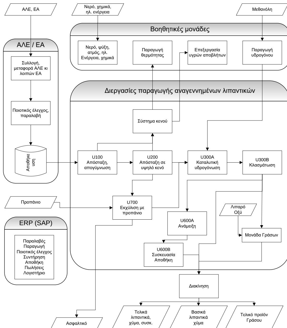
Σχήμα 1-4: Η διεργασία αναγέννησης της LPC
